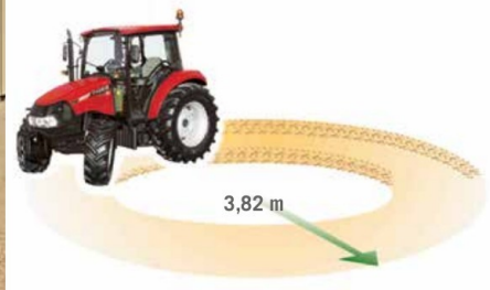
Wenderadius von 3,82 m (Farmall 55 C - 75 C) bzw. 4,33 m (Farmall 85 C - 115 C).
