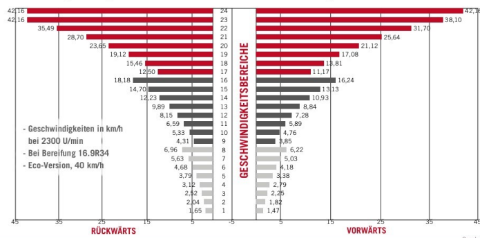
Geschwindigkeitsdiagramm für 24/24-Getriebe mit 2 Lastschaltstufen, 40 km/h ECO
